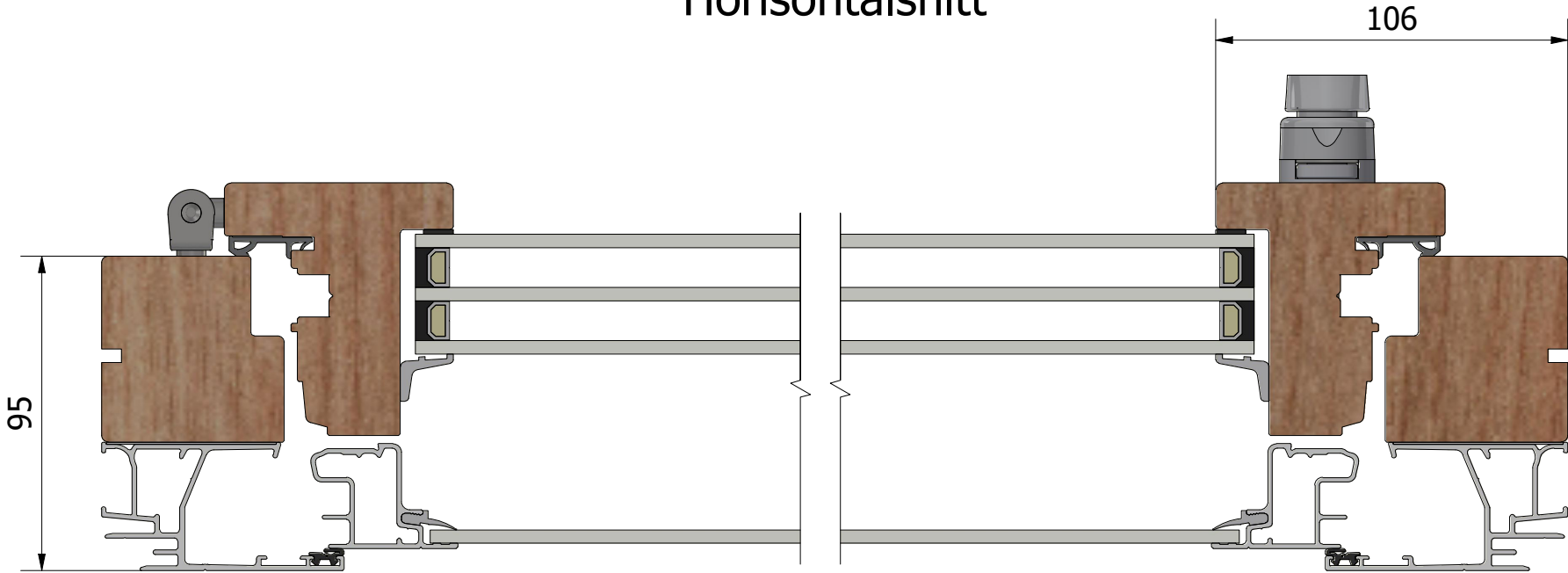
Horizontalsnitt
