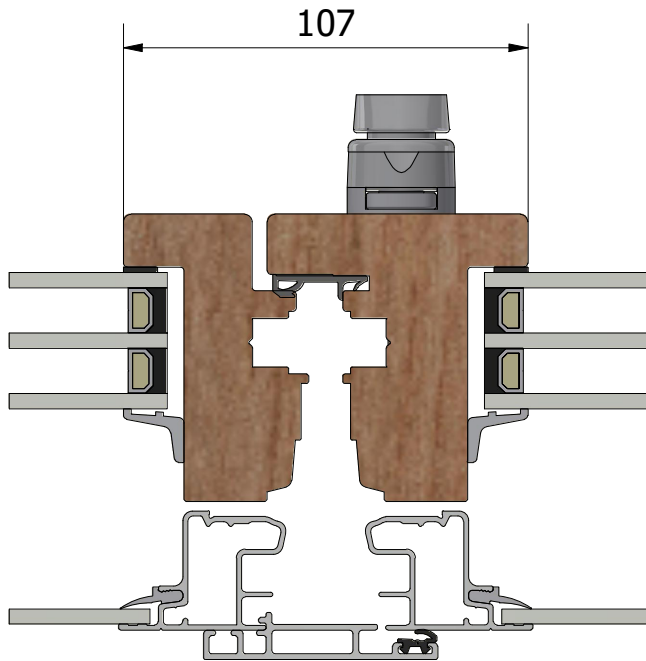
Mötesbåge
