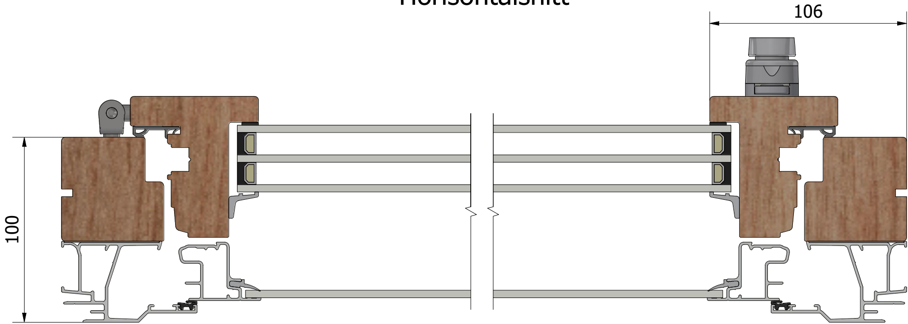
Horizontalsnitt
