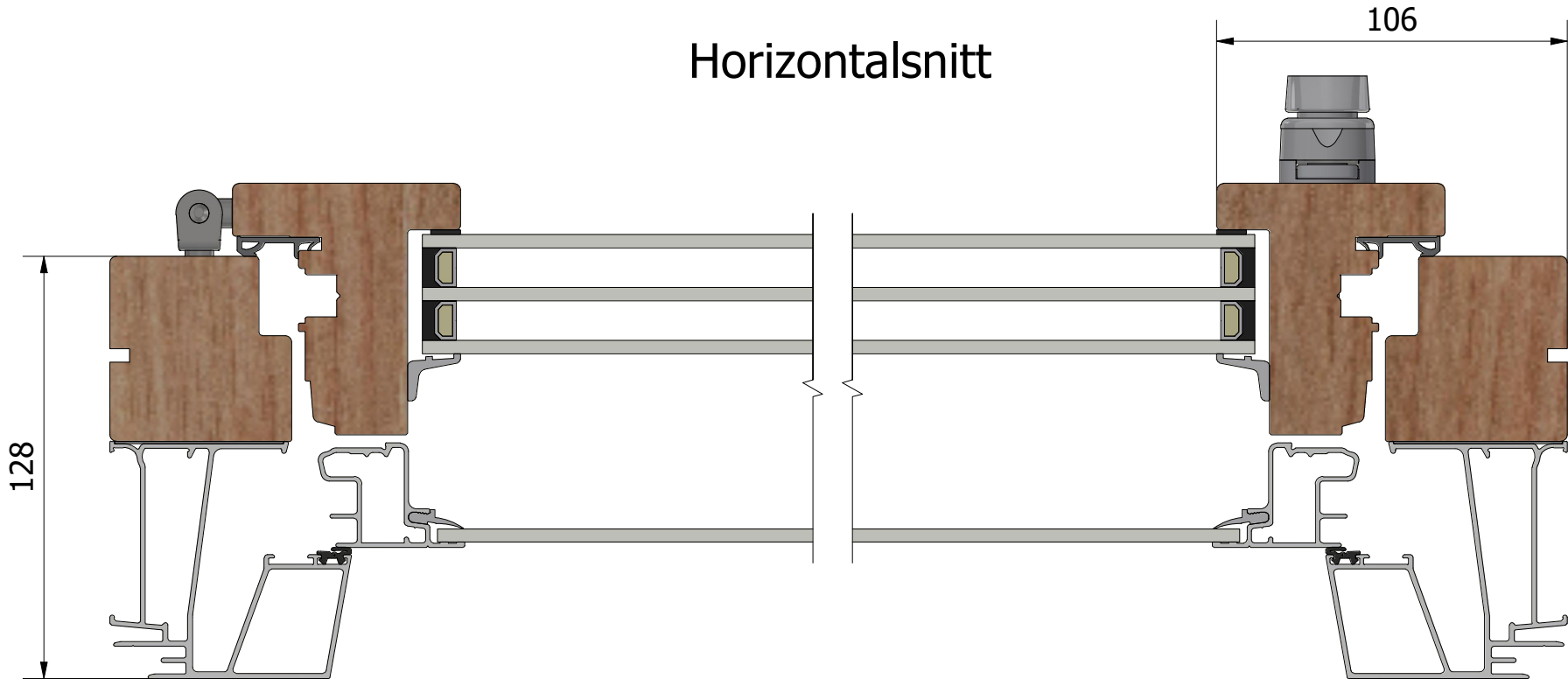
Mötesbåge
