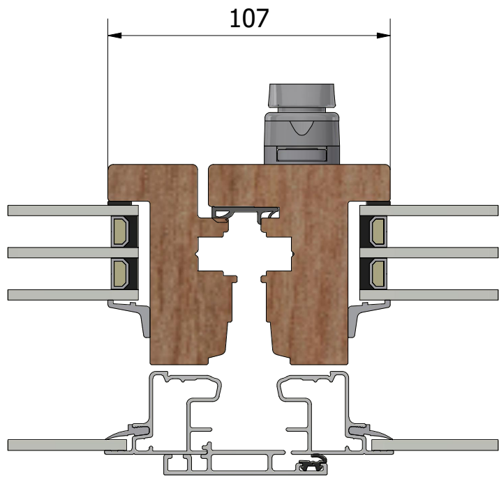
Mötesbåge
